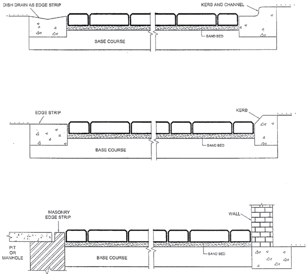
Fig. 8 Edge Restraints
